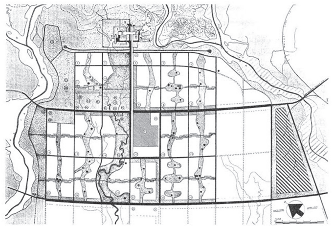
Le Corbusiérovnávrh urbanistického riešenia
