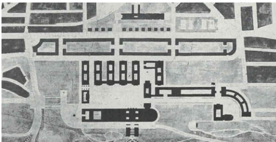
Kamil Roškot umiestnil dominantnú budovu parlamentu v predĺžení osi Čechovho mostu. Uprostred kompozície budov je piazzeta obklopená snemovňou a ďalšími verejnými stavbami. 1928. Zdroj: [7]
