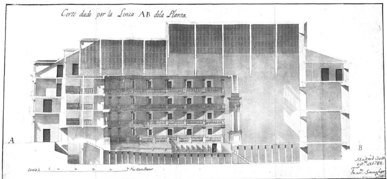
Front and longitudinal section of the Coliseo de los Caños del Peral (Francisco Sánchez, 1788. In "Revista de Archivos y Bibliotecas", 1926. Biblioteca Nacional de España, Madrid)
